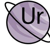
Uranus
