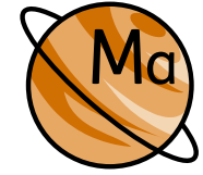
Mars
