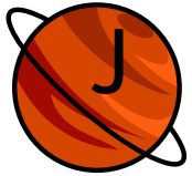
Jupiter
